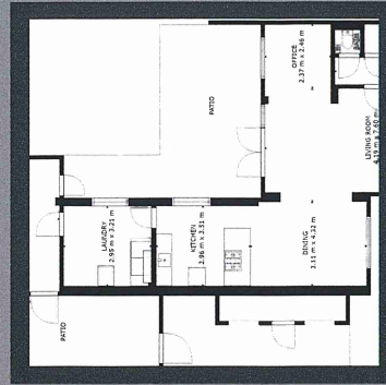
Schematische plattegronden
